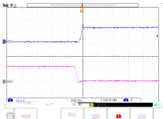
Figure 15. SW edge
